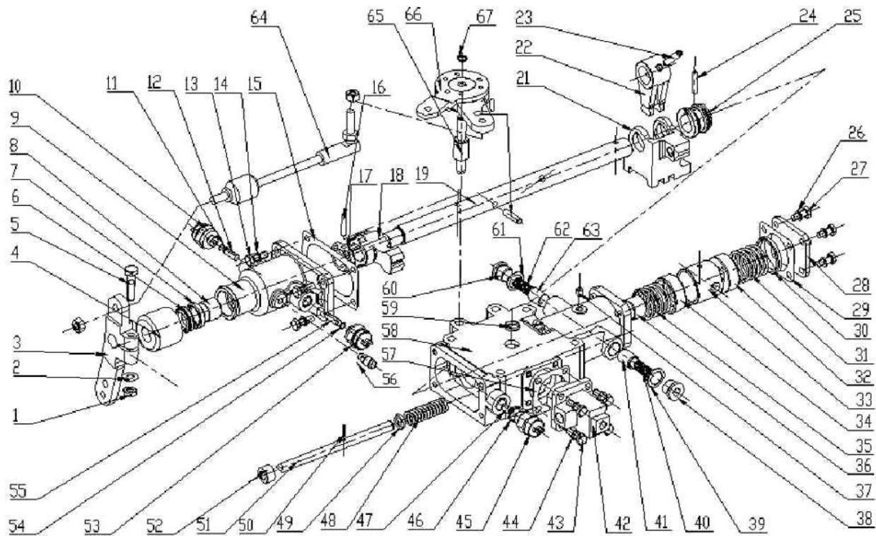
小盖组件（双杆）
