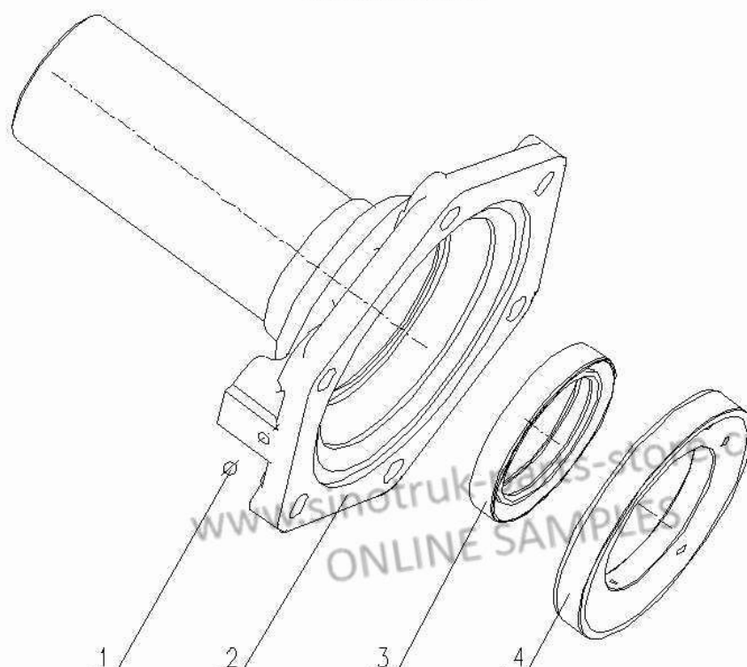
输入轴端盖及导油环
