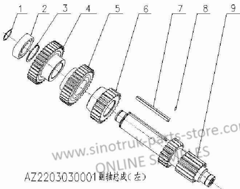
副轴总成（左）
