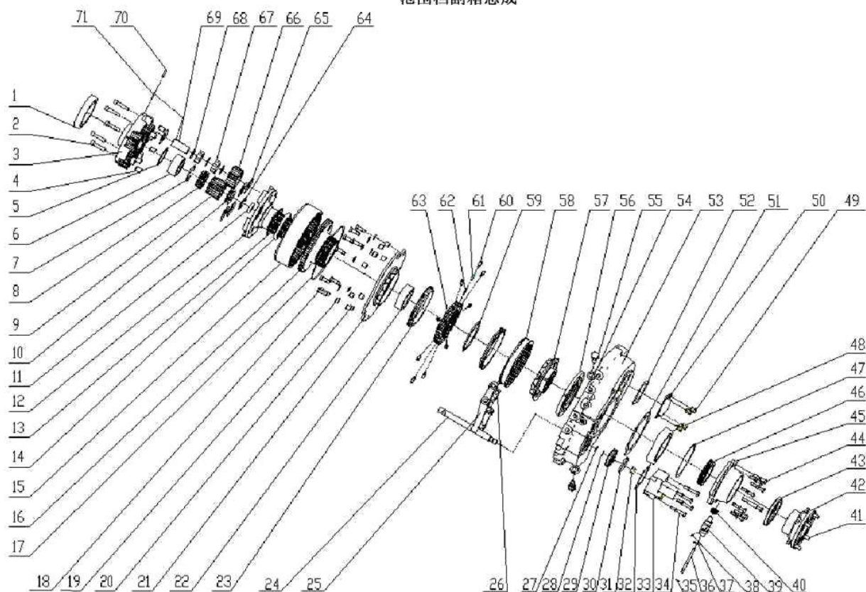
范围档副箱总成
