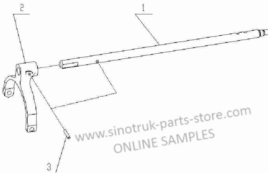
插分档拨叉轴总成
