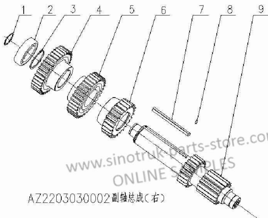
副轴总成（右）
